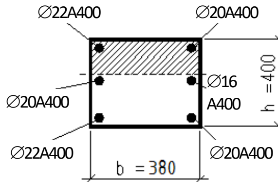
Рисунок 3 – Схема перерізу надкранової частини при розрахунку із площини згину
