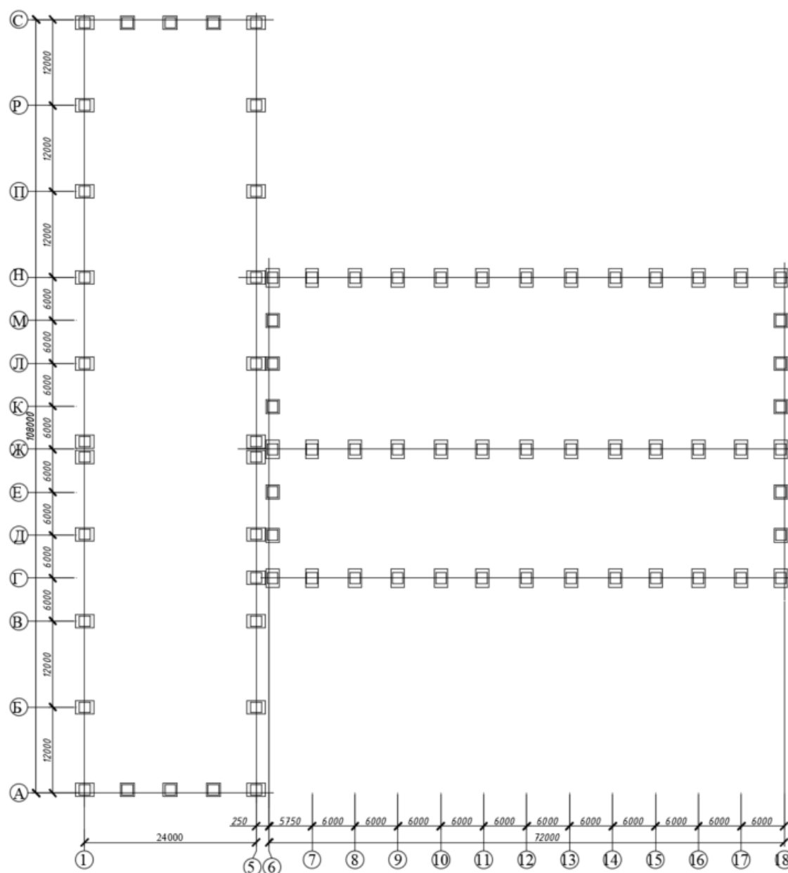
Рисунок 1 – План фундаментів
