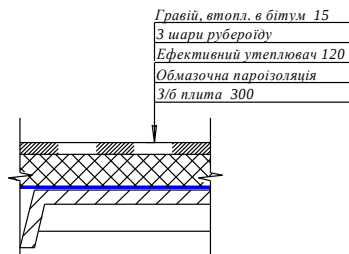
Рисунок 3 – Фрагмент покрівлі
