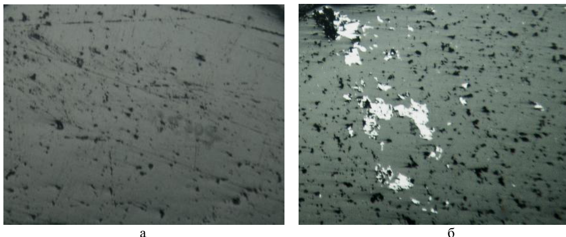
Рис. 4. Особенности структуры и минерального состава нерудных частиц, присутствующих в составе агломерационной руды.
