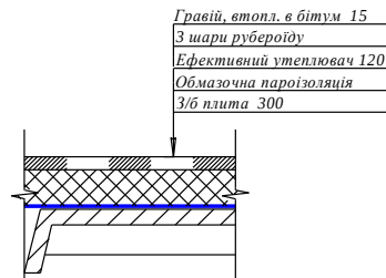
Рисунок 3 – Фрагмент покрівлі
