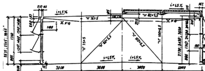
Рисунок 4 – Ліхтар при ширині 12 м
