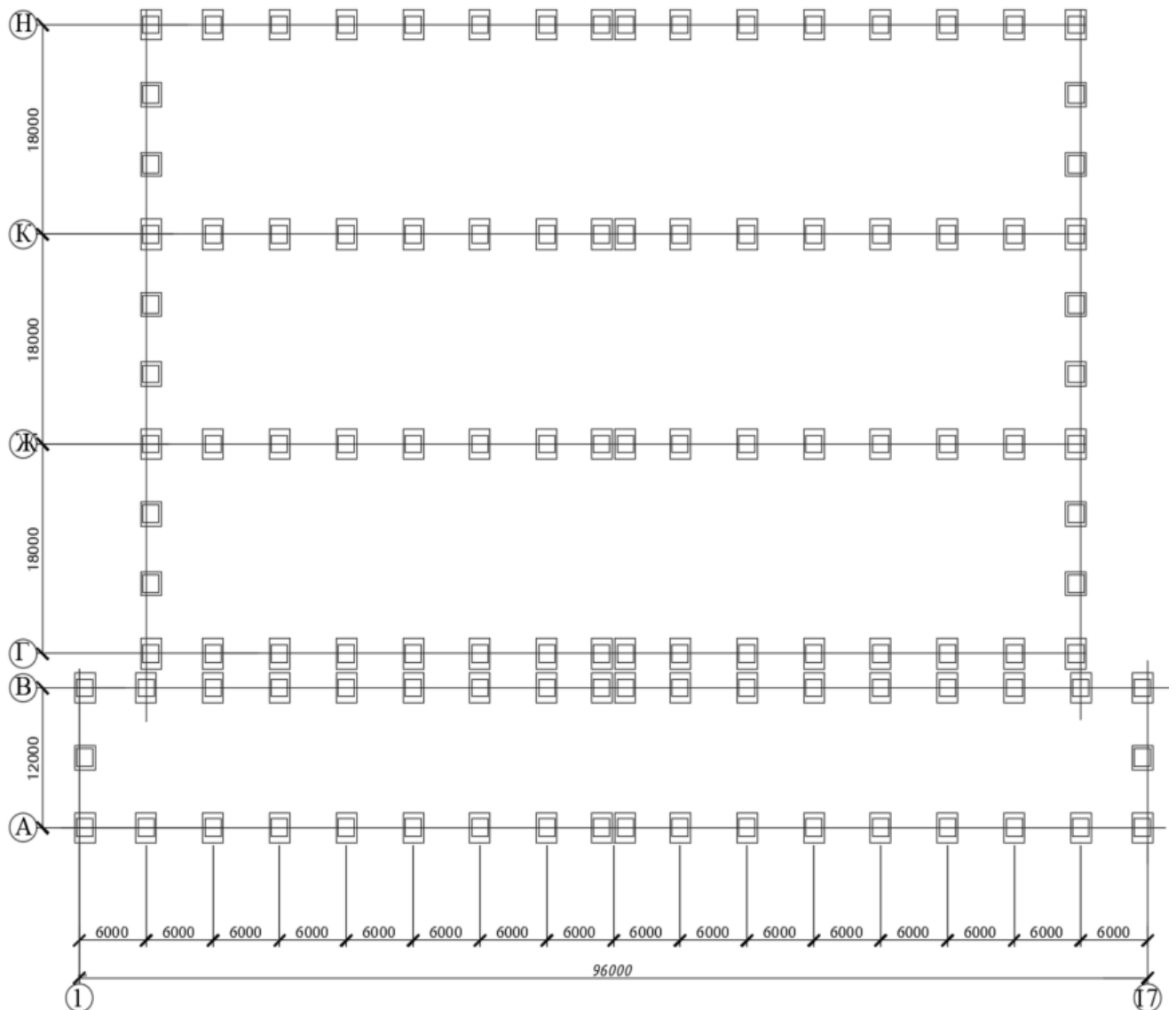
Рисунок 1 – План фундаментів
