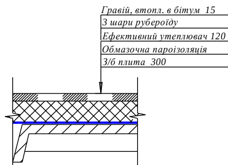
Рисунок 3 – Фрагмент покрівлі
