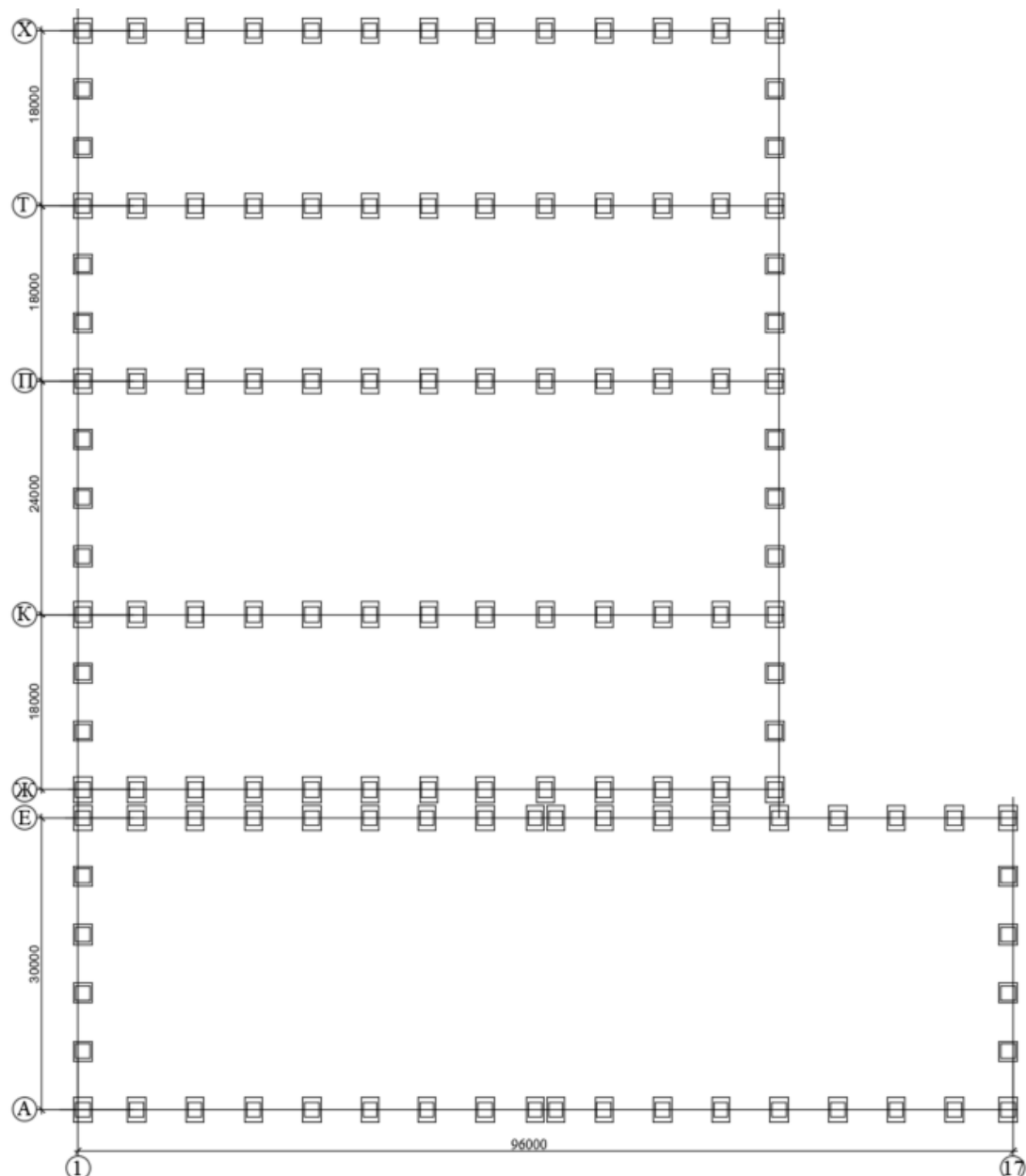
Рисунок 1 – План фундаментів
