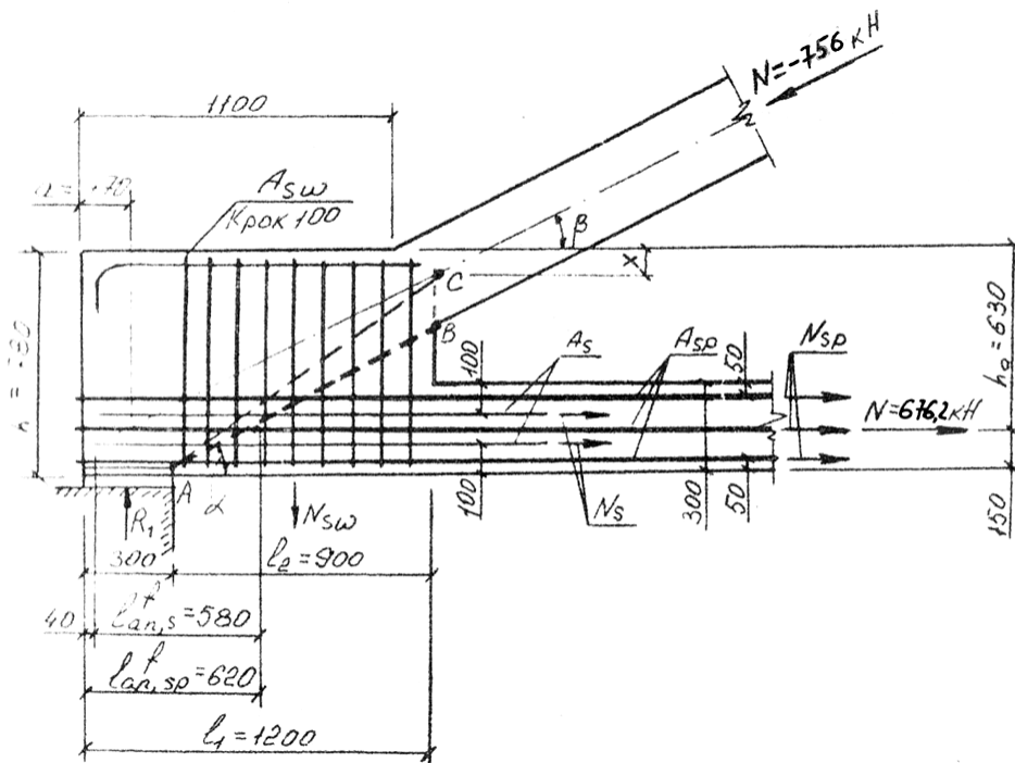
Рисунок 2 – Опорний вузол
