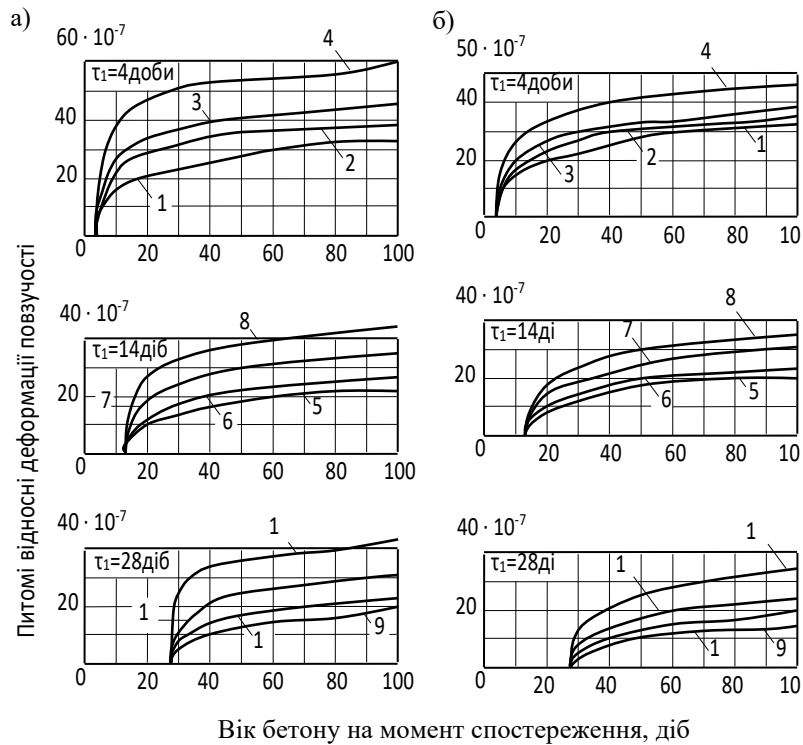
Рис. 1. Експериментальні криві питомих деформацій повзучості при різних рівнях сталих напружень стискання з врахуванням (а) та без врахування (б) деформацій, що натікають за час витримки при навантаженні:
