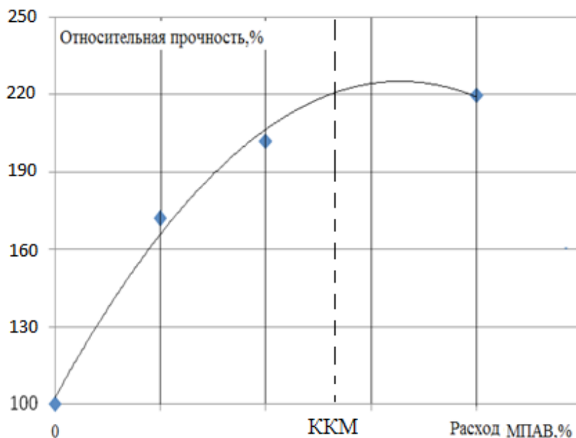
Рис. 1. Влияние МПАВ на прочность RPC
