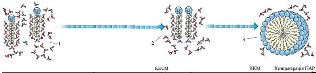
Рис. 2. Зміни структури системи «вода – колоїдна ПАР (МПАР)»: 1 – вільні молекули пар; 2 – димери молекул МПАР; 3 – міцела
