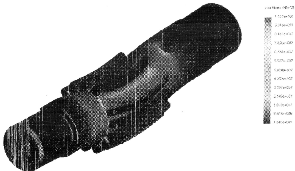
Рисунок 2. Пример расчета напряжений вала первой ступени редуктора вращателя бурового става станка
