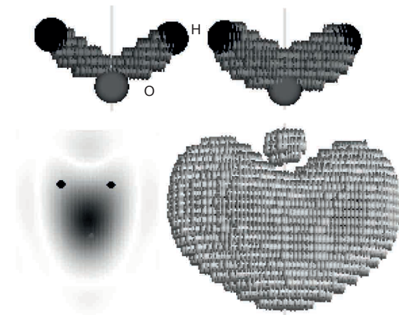
Рис. 3. Просторові розподіли густини валентних електронів в молекулі води: (зліва направо, згори вниз) в інтервалі 1,0–0,9 від максимального значення, в інтервалі 0,9–0,8, переріз просторових розподілів густини валентних електронів, просторовий розподіл в інтервалі 0,2–0,1
