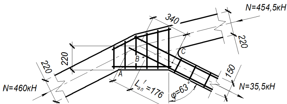
Рис. 2.2.5.2 – Розрахункова схема 1-го проміжного вузла верхнього поясу
