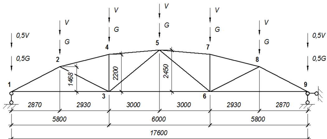
Рис. 2.2.2.1 – Розрахункова схема ферми
