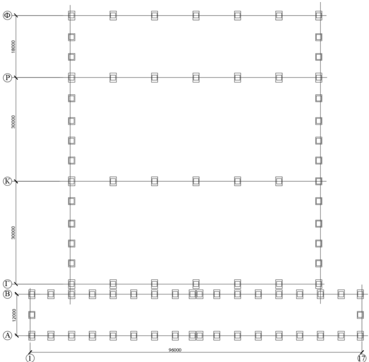
Рисунок 1 – План фундаментів
