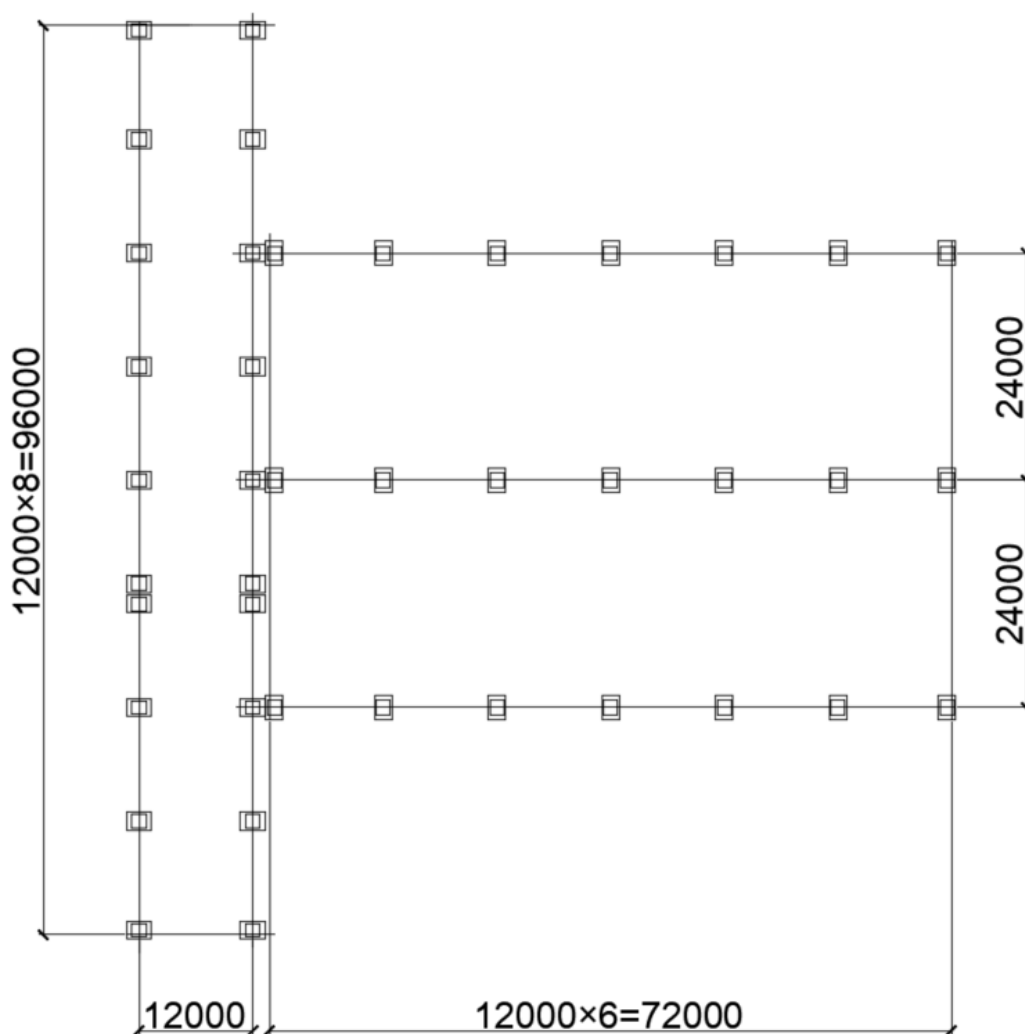
Рисунок 1 – План фундаментів
