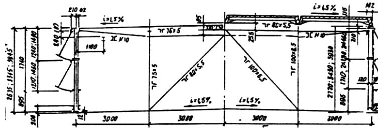
Рисунок 4 – Ліхтар при ширині 12 м
