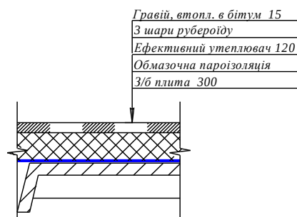
Рисунок 3 – Фрагмент покрівлі
