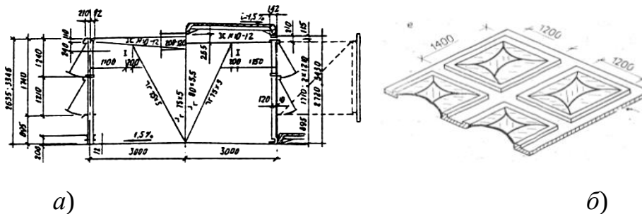
Рисунок 4 – Ліхтарі: а – при ширині 6 м; б – зенітний
