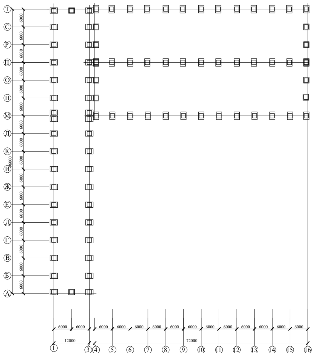
Рисунок 1 – План фундаментів
