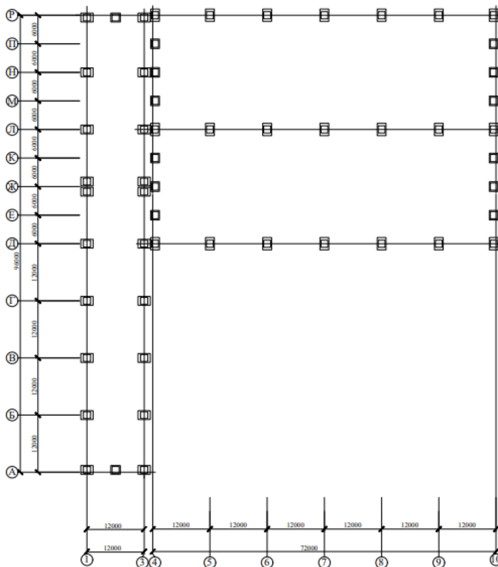
Рисунок 1 – План фундаментів
