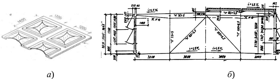
Рисунок 4 – Ліхтарі: а – zenітний; б – при ширині 12 м
