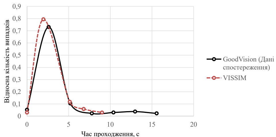
Рис.2.10. Залежність відносної кількості випадків від часу проходження маршруту на перехресті після калібрування.
