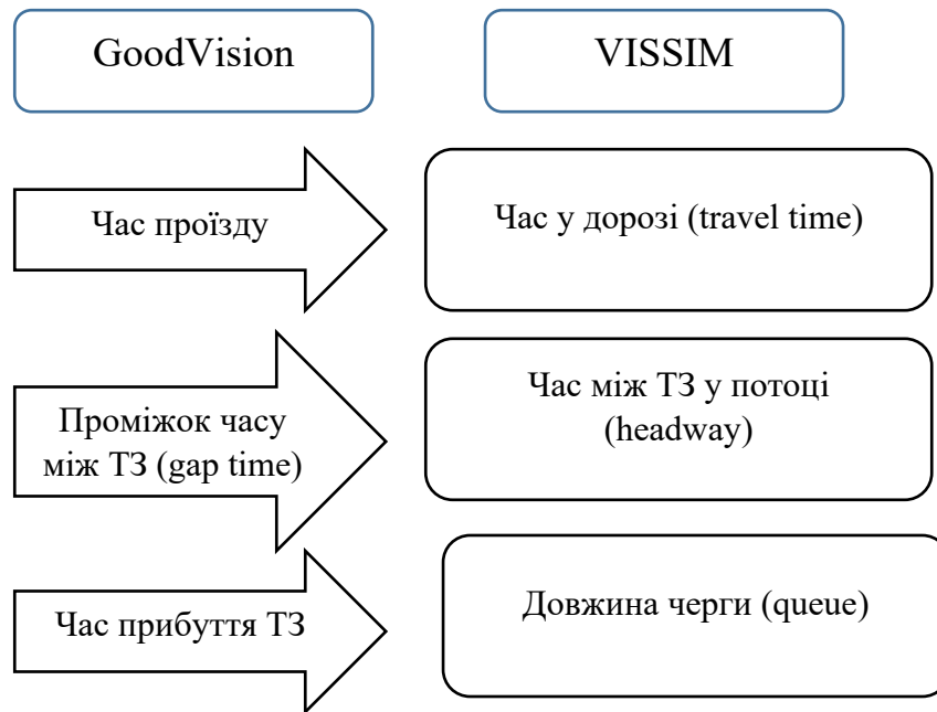
Рис.2.2. Вихідні параметри GoodVision та відповідні ним показники калібрування VISSIM.
