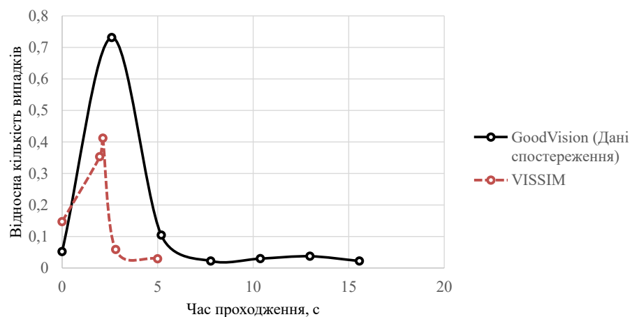
Рис.2.8. Залежність відносної кількості випадків від часу проходження маршруту на перехресті до калібрування.
