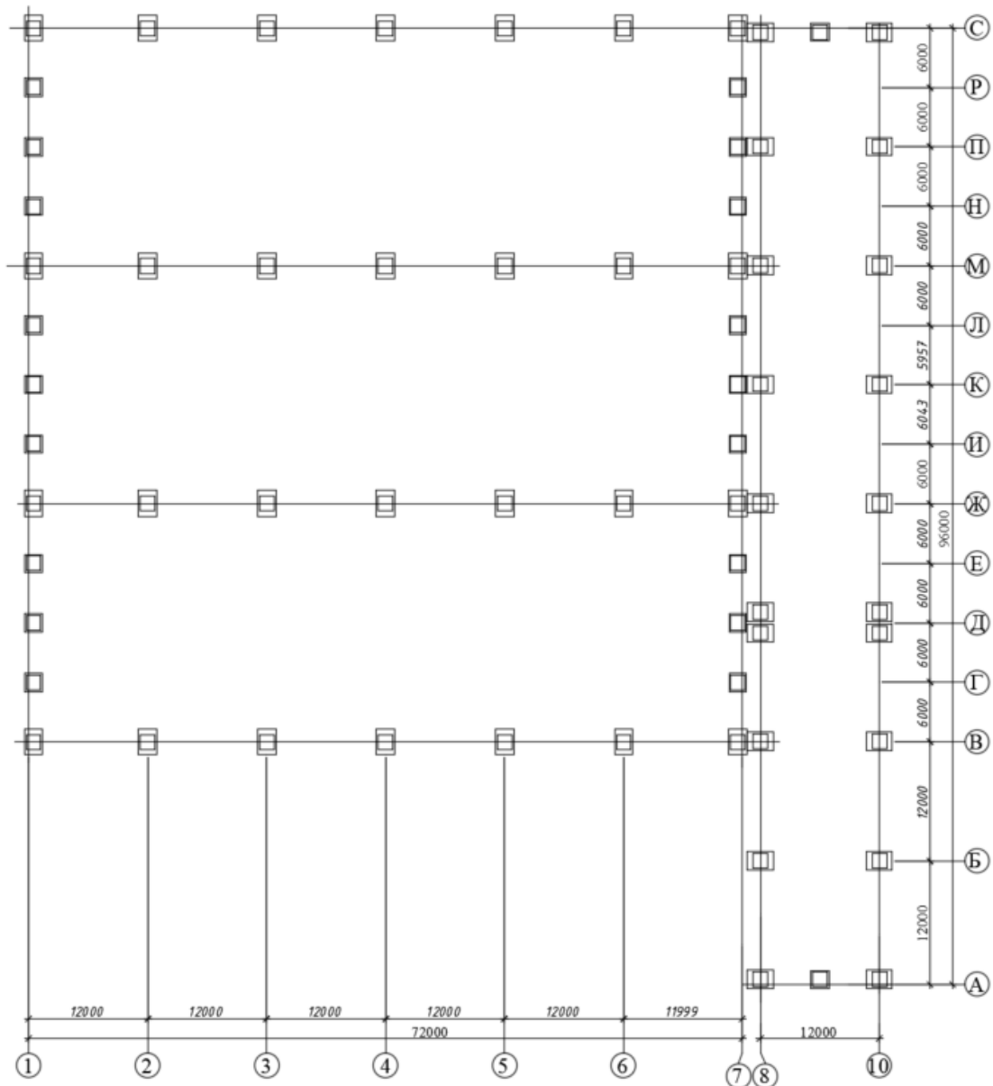
Рисунок 1 – План фундаментів
