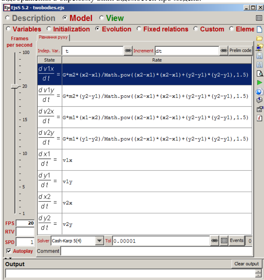
Рис. 3.24. Визначення системи рівнянь руху
