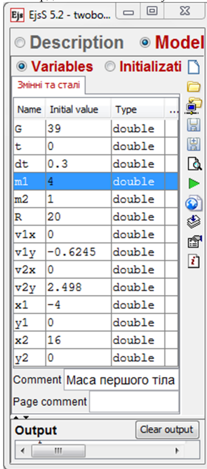
Рис. 3.23. Визначення параметрів (змінних та сталих) моделі
