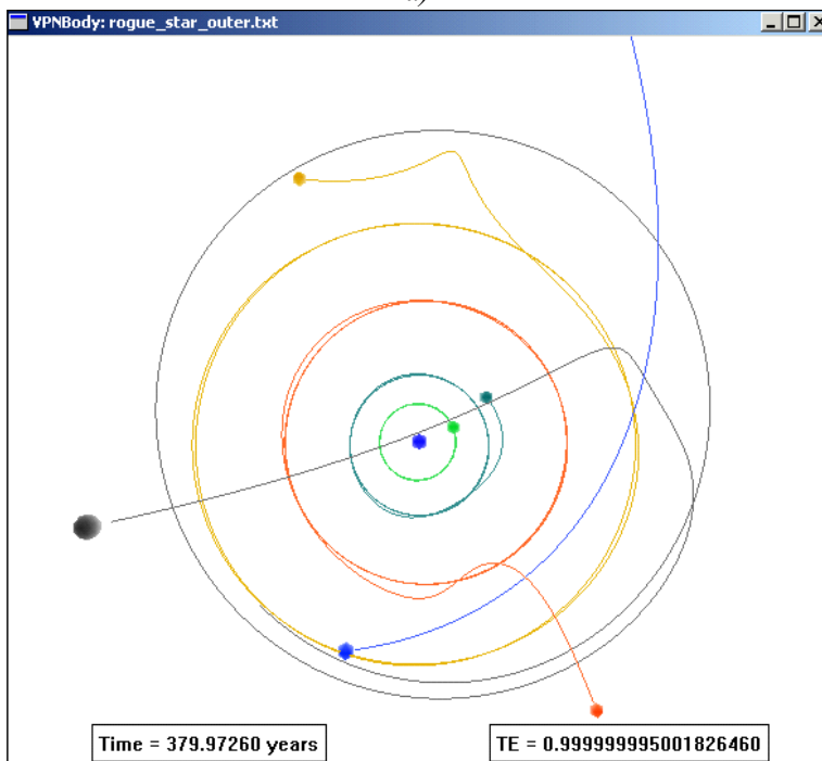
Рис. 3.7. Фрагмент опису комп'ютерної моделі процесу вторгнення в Сонячну систему блукаючої зірки масою в 1,5 маси Сонця у ПЗ моделювання сонячно-подібних систем VPBody (а) та результати моделювання (б)
