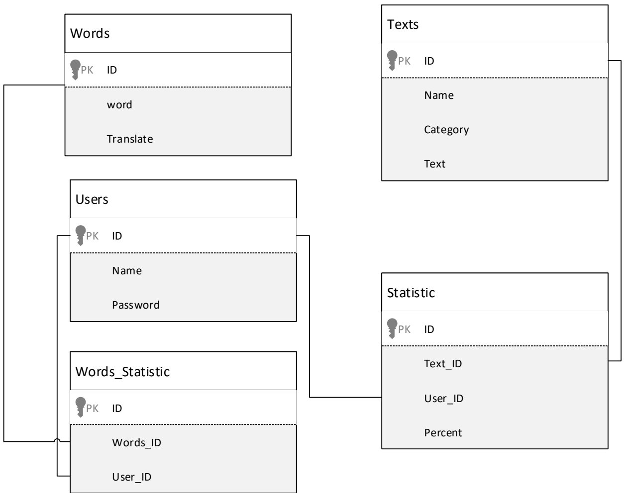
Рисунок 2.8 – ERD діаграма бази даних тренажеру з англійської мови на прикладі художніх текстів
