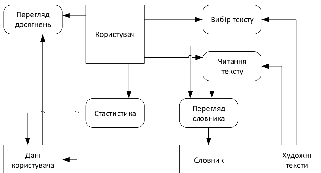
Рисунок 2.2 – Детальна діаграма потоків даних тренажера з англійської мови на прикладі художніх текстів
