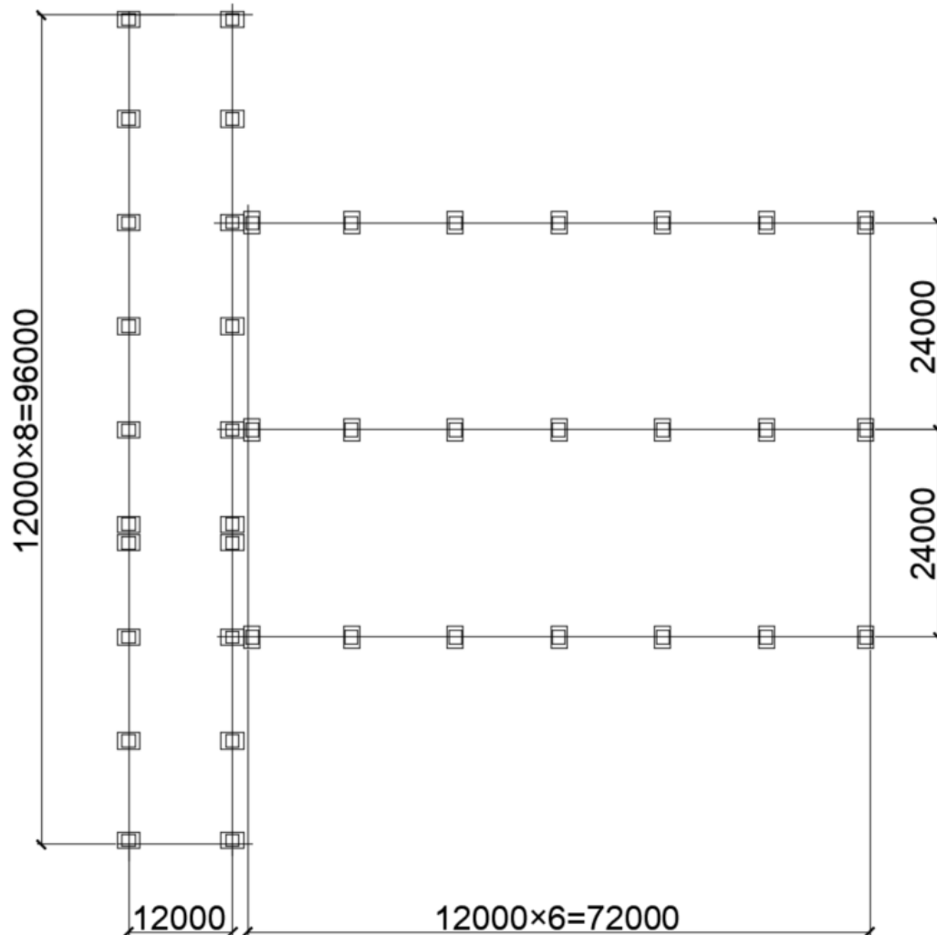
Рисунок 1 – План фундаментів
