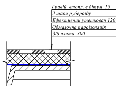
Рисунок 3 – Фрагмент покрівлі
