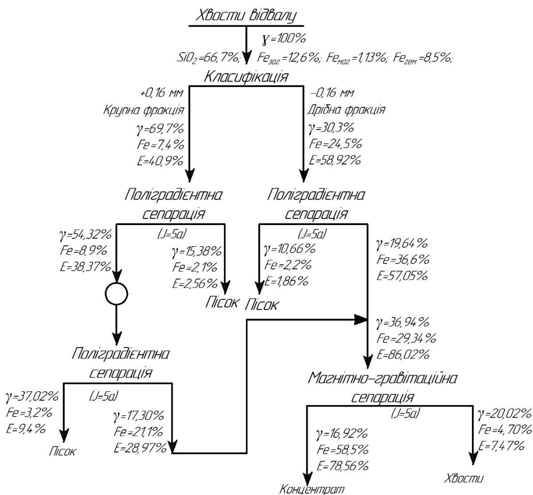
Рис. 1. – Рекомендована схема збагачення відходів
