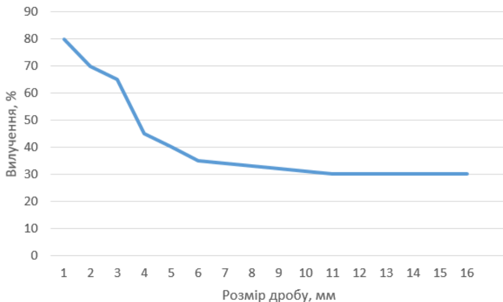
Рис. 2 – Залежність вилучення від розміру куль
