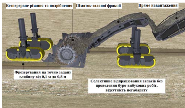
Рис. 1. Конструкція та принцип дії фрезерного комбайна
