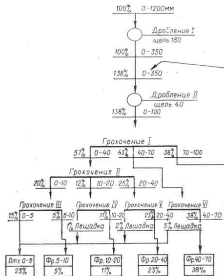
Рис. 1. Технологическая схема фабрики нерудных материалов ГОКа
